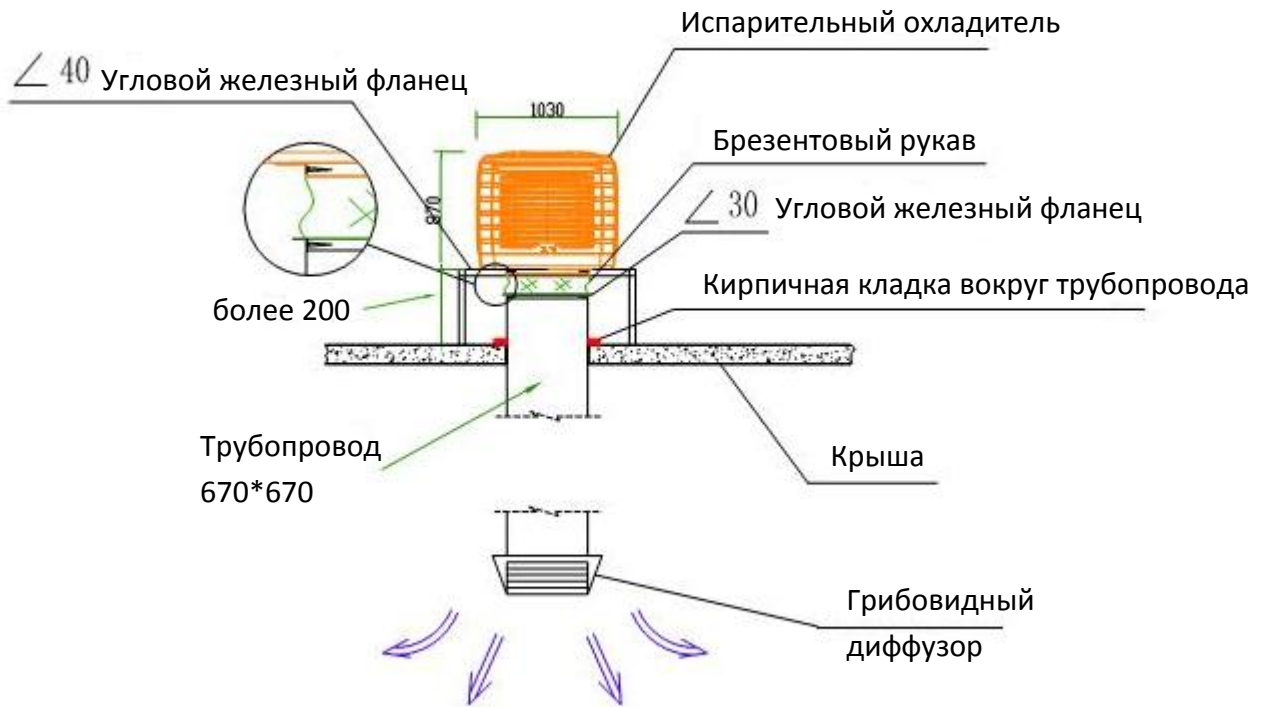
Схема установки испарительного охладителя на цементной крыше
