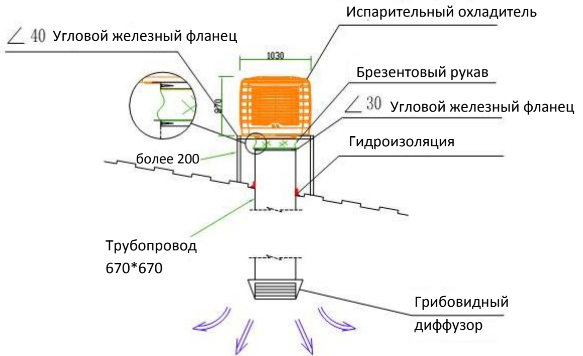
Схема установки испарительного охладителя на крыше (металл, стеклочерепица)
